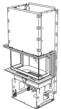
Einbaurahmen B, plan
